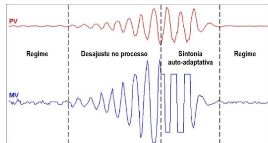
Figura 12 - Ejemplo de una sintonía auto-adaptativa
