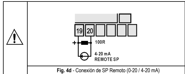
Fig. 4d - Conexión de SP Remoto (0-20 / 4-20 mA)
