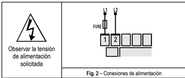
Fig. 2 - Conexiones de alimentación
