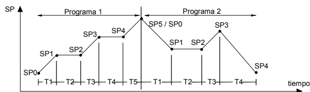
Fig. 11 - Ejemplo de programa 1 e 2 "linkados" (interconectados)
