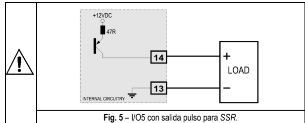
Fig. 5 - I/O5 con salida pulso para SSR.
