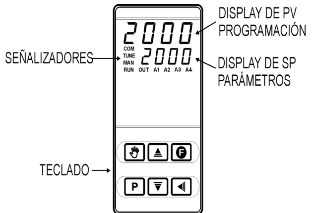
Fig. 8 - Identificación de las partes del panel frontal
