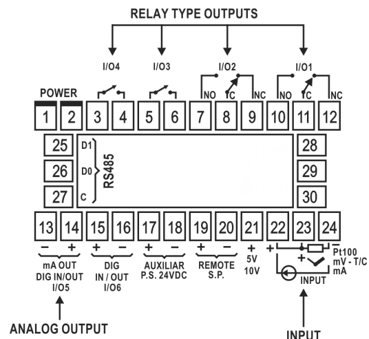
Fig. 1 - Conexiones del panel trasero.
