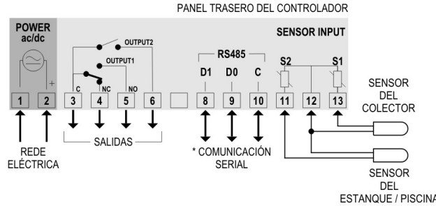
Fig. 1 – Conexiones mostradas en la etiqueta del controlador
